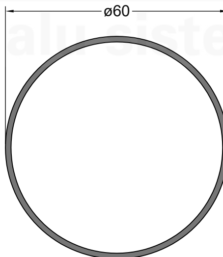
12663 0.744 Kg/m ACOPLE ROTULA CAÑO Ø 60 mm.
