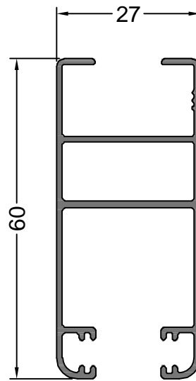
13237 0.657 Kg/m CORREDIZA HOJA JAMBA REFORZADA
