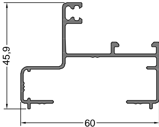
13172 0.656 Kg/m PAÑO FIJO/ABRIR MARCO
