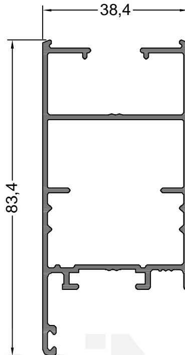
13221 0.985 Kg/m PUERTA HOJA
