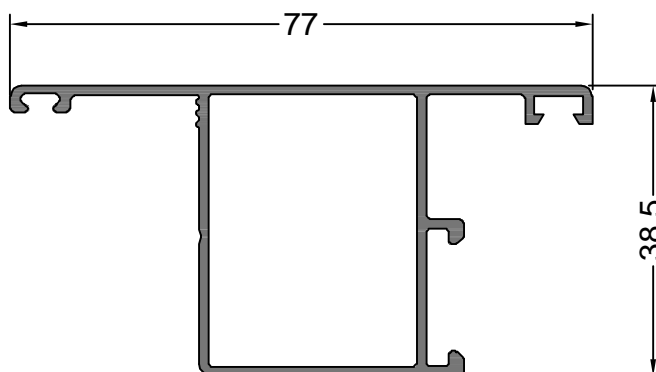
13560 0.714 Kg/m DESPLAZABLE HOJA
