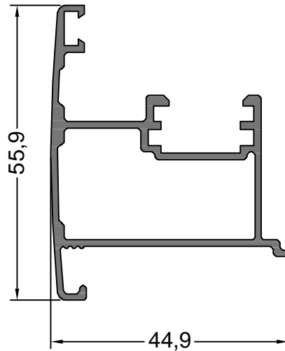
13170 0.729 Kg/m ABRIR ENCUENTRO 2 HOJAS
