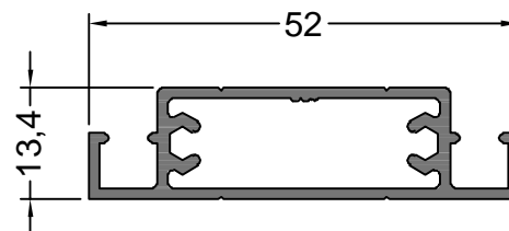
11241 0.506 Kg/m CORREDIZA MOSQUITERO TRAVESAÑO
